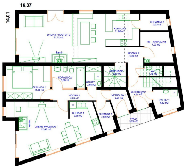
PRITLIČJE
