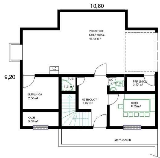
KLET
