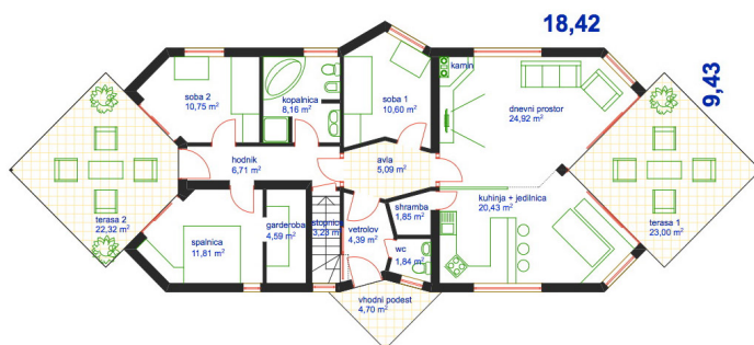
PRITLIČJE
