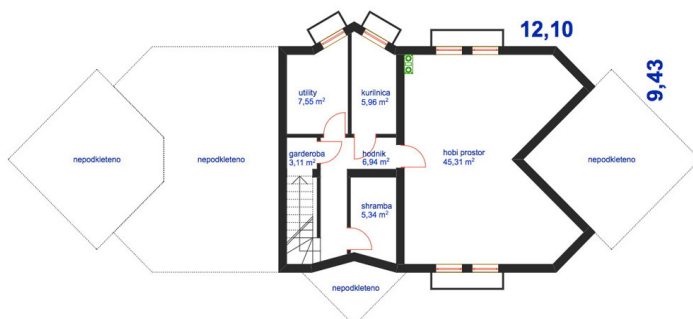
KLET
