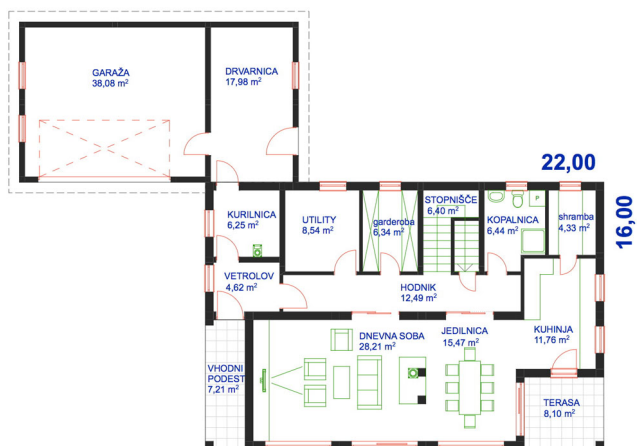
PRITLIČJE
