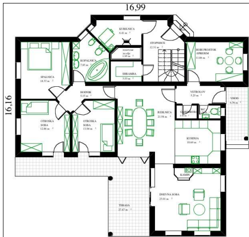
PRITLIČJE
