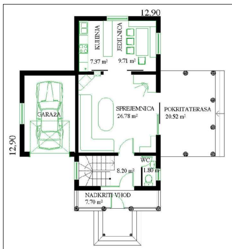
PRITLIČJE
